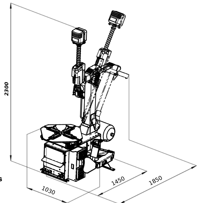
Dimensiones TC47L
